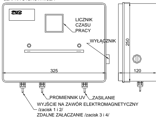
SZAFKA STEROWNICZA
